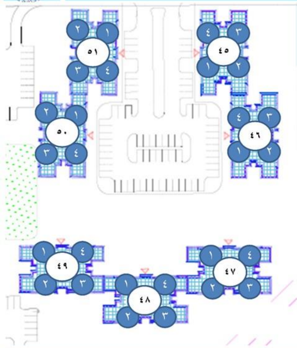
الموقع العام - سكن مصر الواجهة الشرقية - عمارات ٤٥ حتى ٥١
